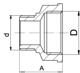
FT221 Redukované pro- dloužení ŠM Extension reduced MF
