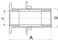
FT220 Prodloužení do bytového jádra Flanged connection for sanitary unit
