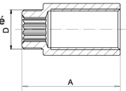
FT219 Prodloužení chromované Chrome flanged connection
