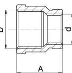
FT218 Nátrubek redukovaný MM Socket reduced FF
