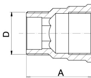
FT216 Prodloužení kované Forged flanged connection
