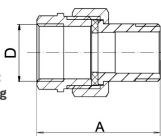
FT209 Topenářské šroubení s plochým těsněním Brass screwed fitting with flat gasket for heating engineering
