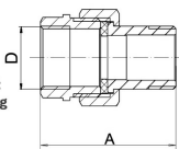
FT209 Topenářské šroubení s plochým těsněním Brass screwed fitting with flat gasket for heating engineering
